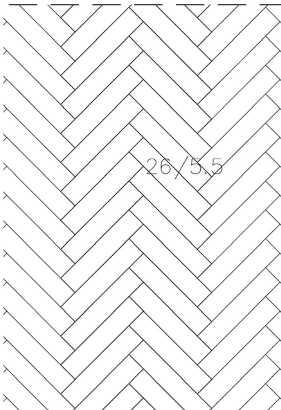
Prostorija 9 - skica završne podne obloge
